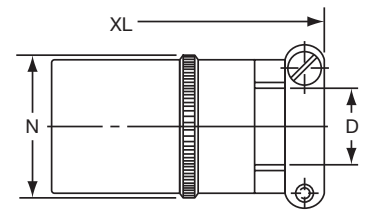
MS3116J-XX-XXX
