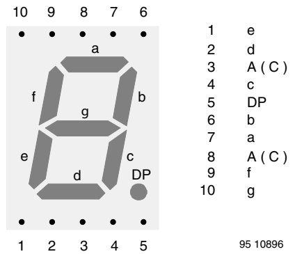
Fig. 7 - TDSR13..
