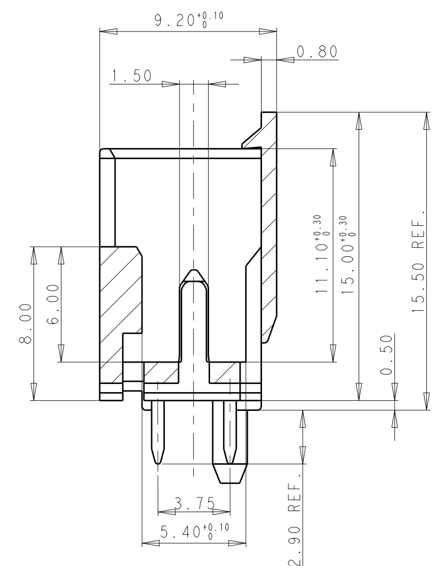
SECTION A-A
