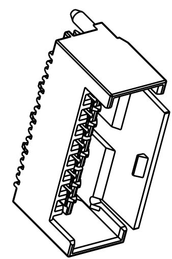
SCALE 2:1
