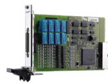
cPCI-7252
