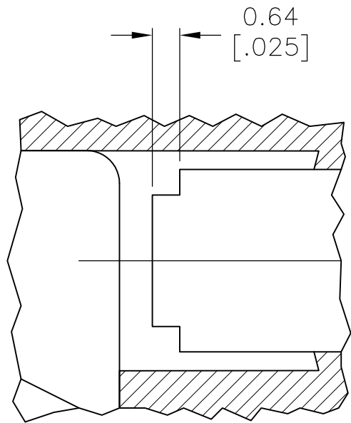
DETAIL Z SCALE 8:1 TYP
