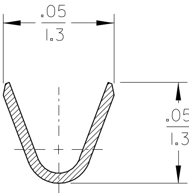
SECTION B-B SCALE: NONE
