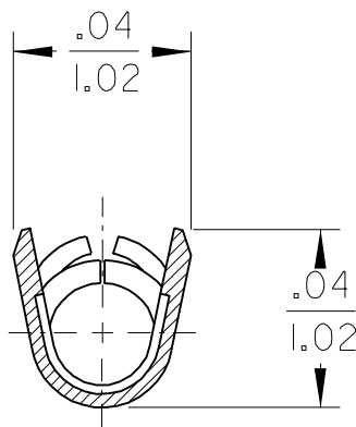
SECTION A-A SCALE: NONE
