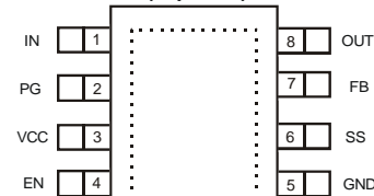
SO-8EP
