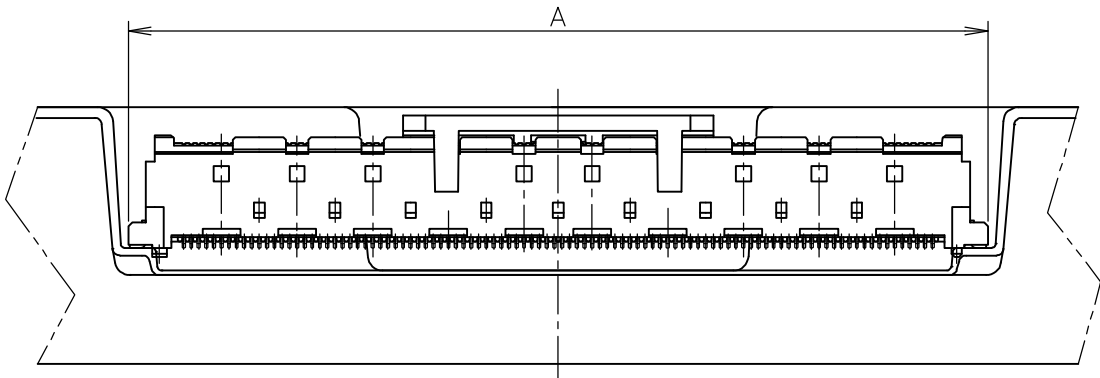
D-D (SCALE 2:1)
