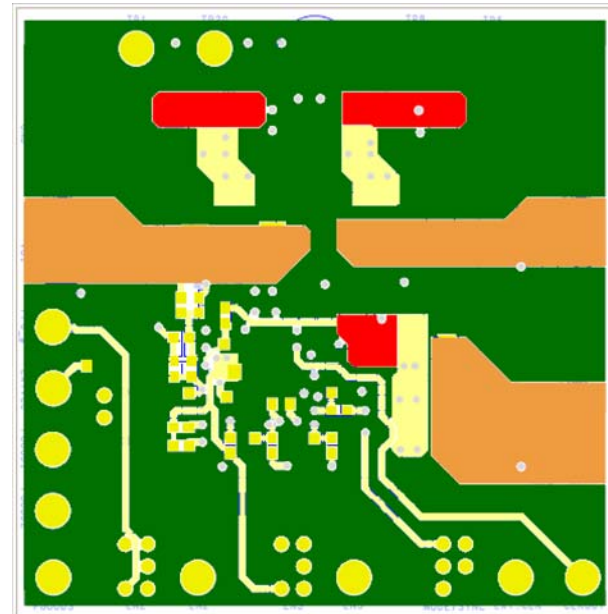
FIGURE 20. BOTTOM LAYER
