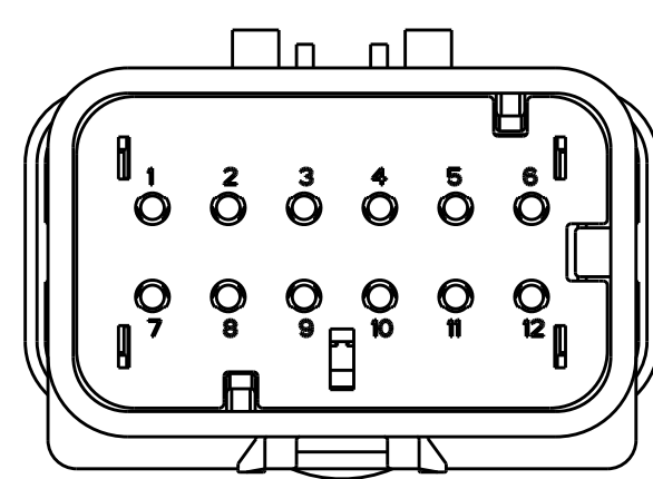
776438-3 SCALE 2:1
