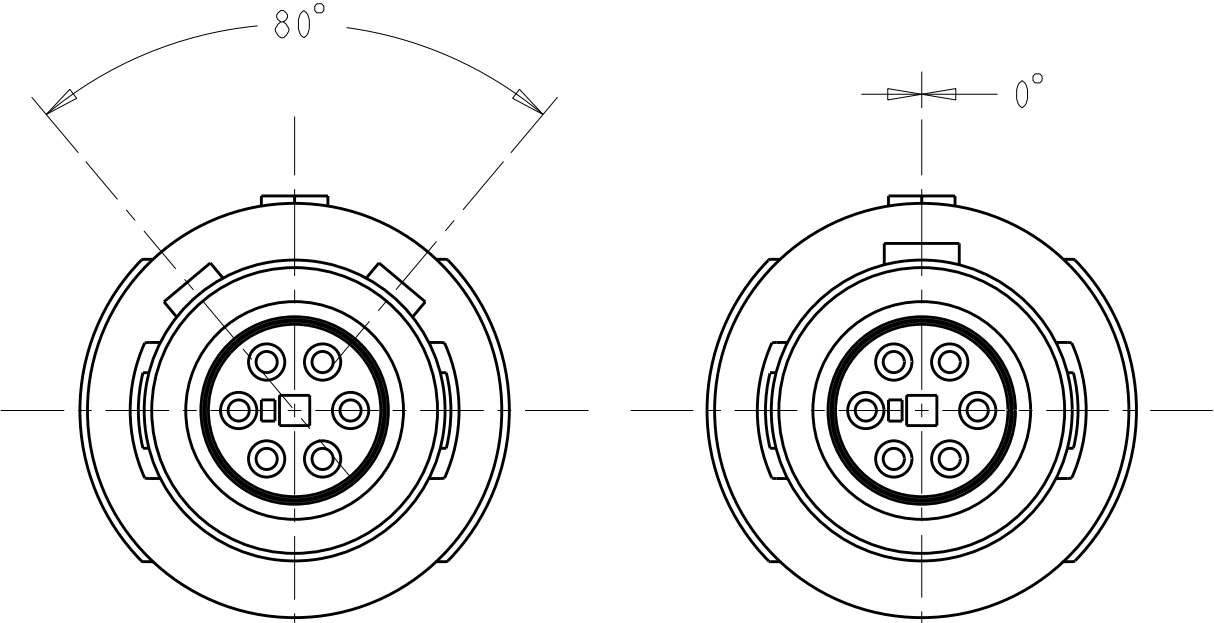
80° KEYING SCALE 4:1
