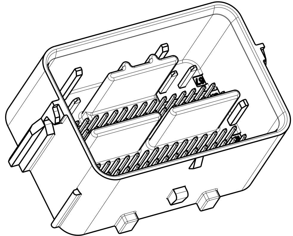
SCALE 2:1
