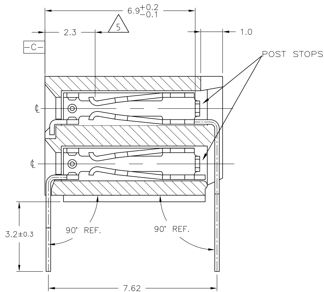
SECTION A-A
