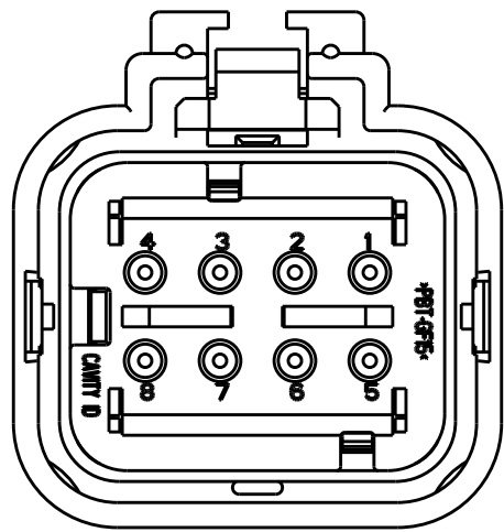
776532-2 (GRAY TPA) SCALE 2:1
