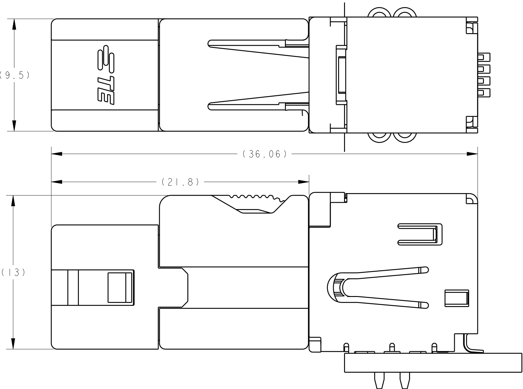
CAP ASSEMBLY & PLUG ASSEMBLY ENGAGEMENT DRAWING キャップアセンブリ & プラグアセンブリ 嵌合図
