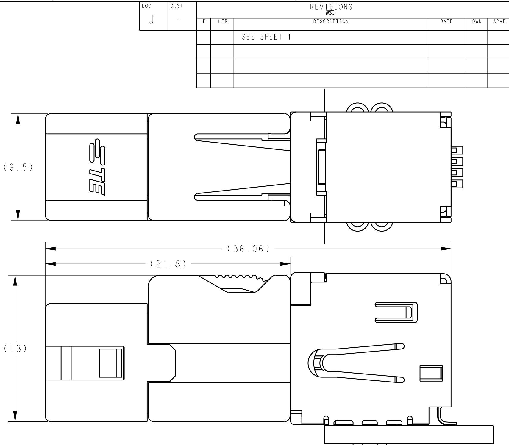
CAP ASSEMBLY & PLUG ASSEMBLY ENGAGEMENT DRAWING キャップアッセンブリ & プラグアッセンブリ 嵌合図
