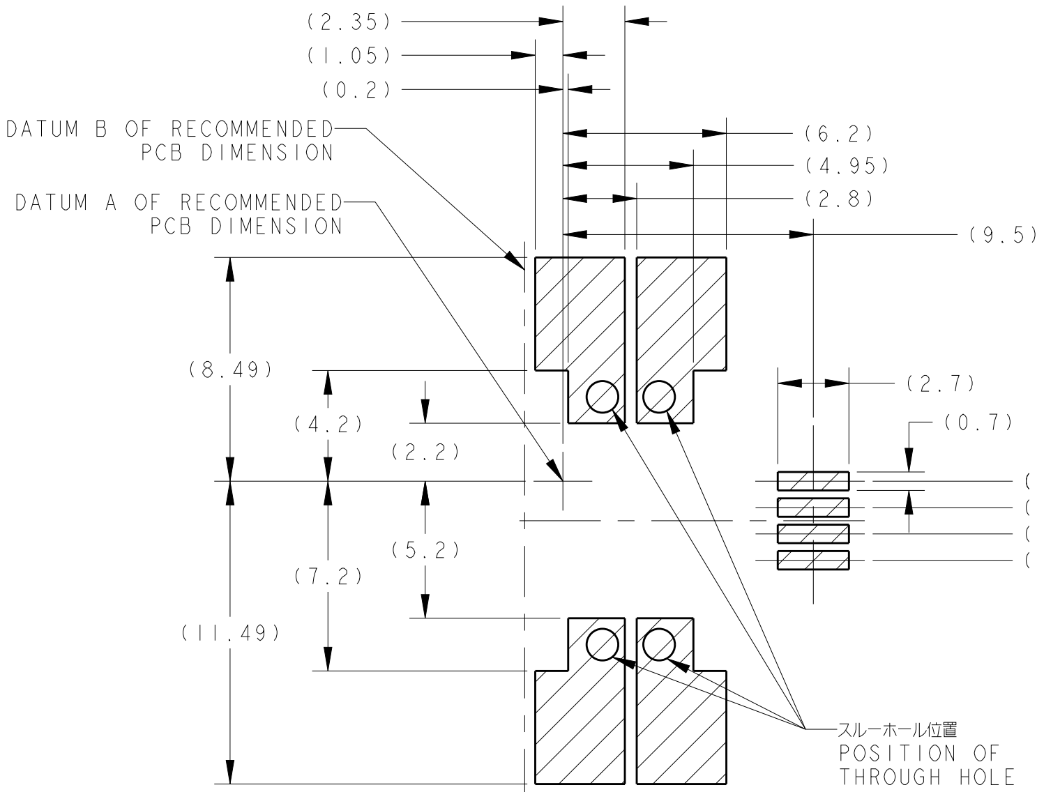
3. メタルマスク寸法 (参考) (t=0.15) METAL MASK DIMENSION (REFERENCE)
