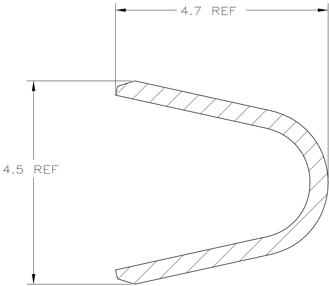
SECTION A-A SCALE 20:1
