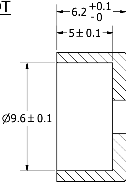
A-A ( 5 : 1 )
