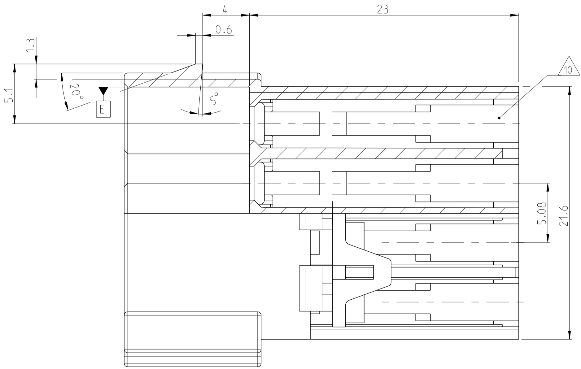
SECTION B-B Schnitt
