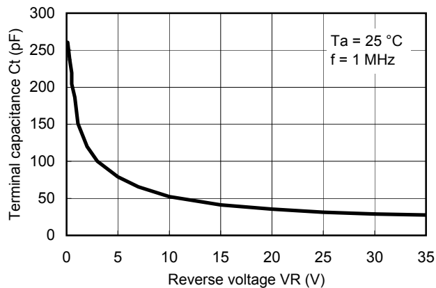
Ct - VR
