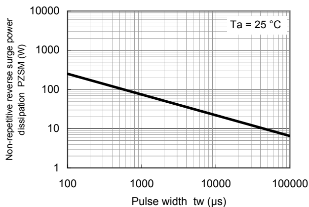
PZSM - tw
