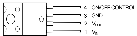
NJM2388F
