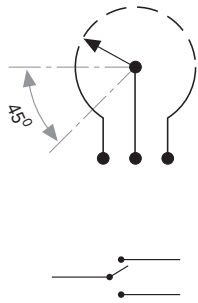
SPDT Switch
