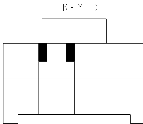
KEYING FOR 2*4 POS.
