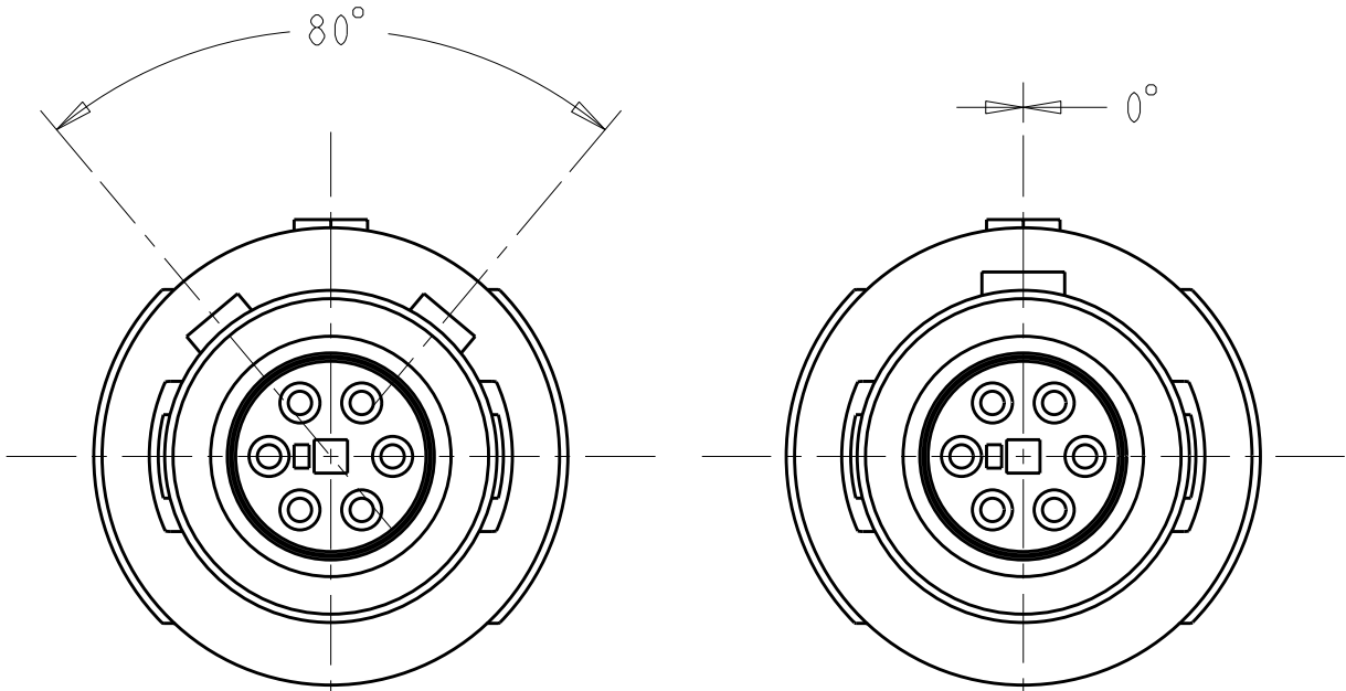
80° KEYING SCALE 4:1
