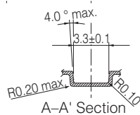
A-A' Section
