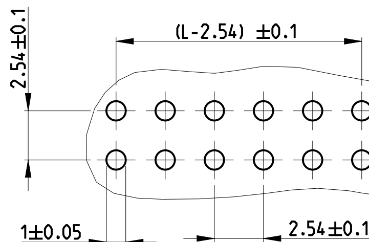
PC BOARD LAYOUT LEITERPLATTENANSCHLUSSBILD
