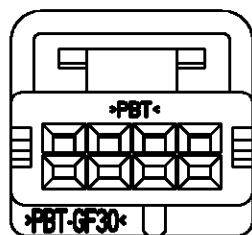
638119-2 SCALE 2:1
