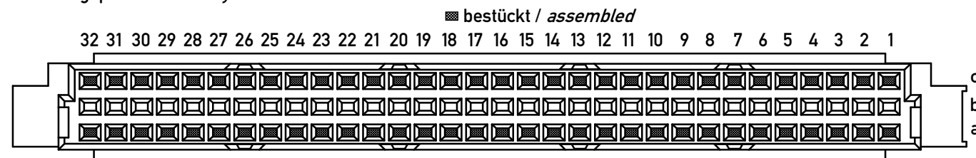
Bestückungsplan / contact layout
