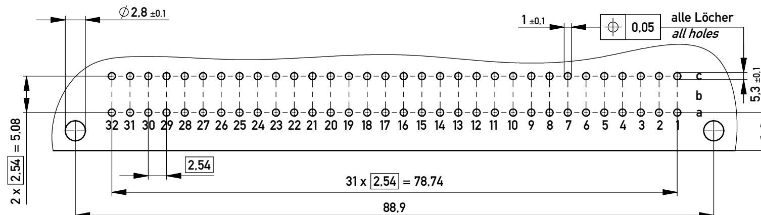
Leiterplatten-Lochbild / PCB drillhole pattern
