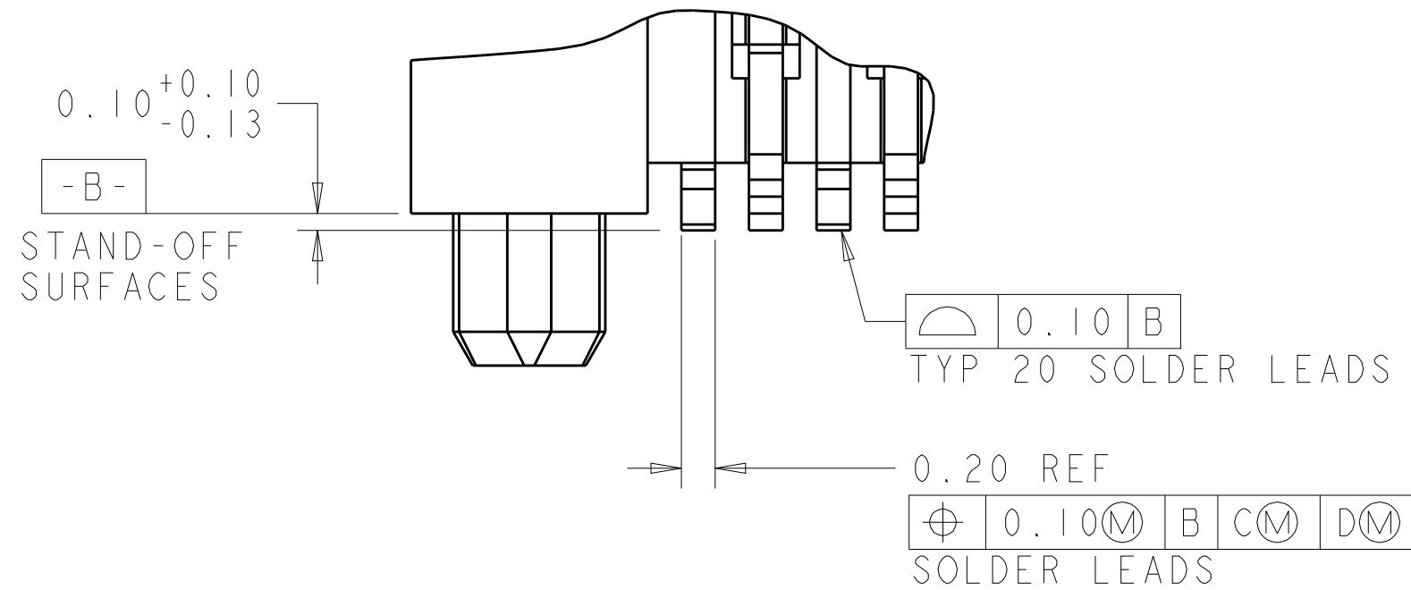
DETAIL H SCALE 25:1
