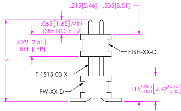
FIG 2 (BKT MACHINE)
