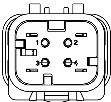
776488-2 SCALE 2:1
