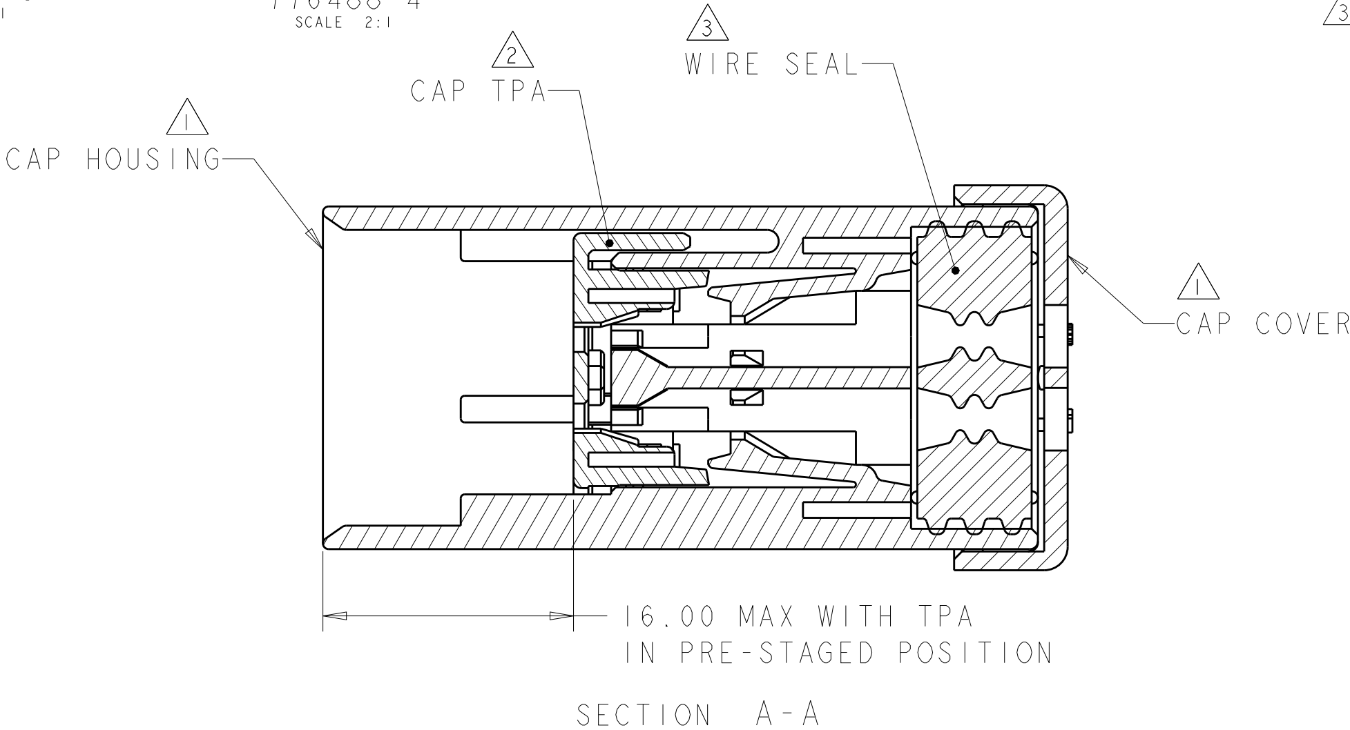
776488-4 SCALE 2:1
