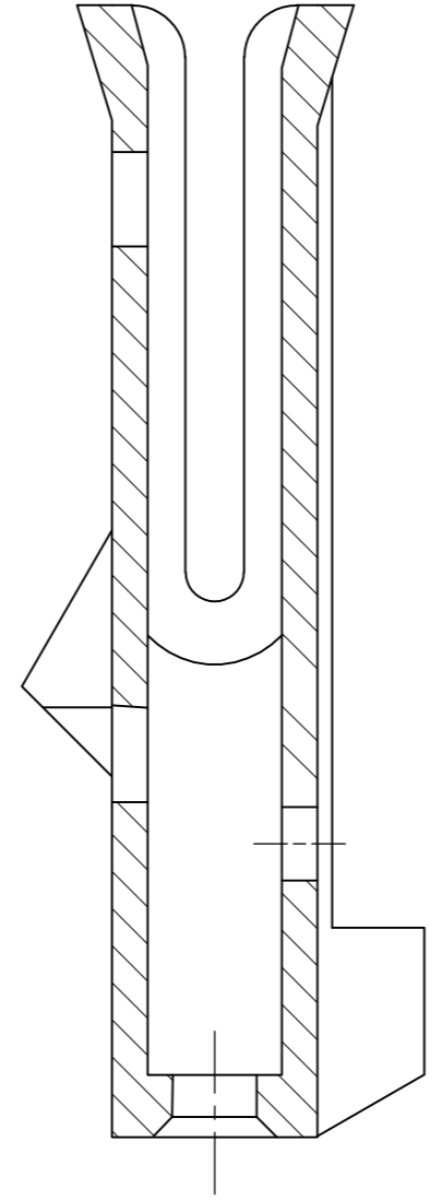
SECTION D-D
