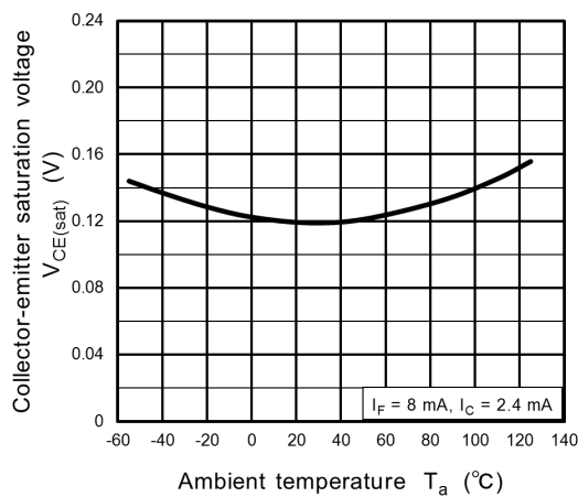
Fig. 11.10 V_{CE(\text{sat})} - T_a
