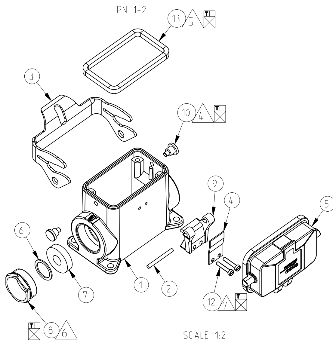
SCALE 1:2
