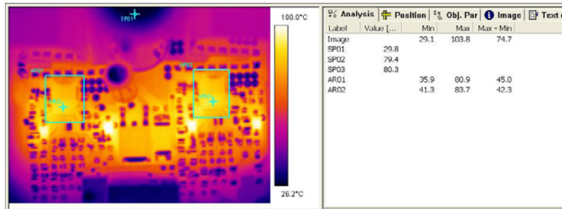
Fig 7 IRAUDAMP15 (Vbus=31V)
