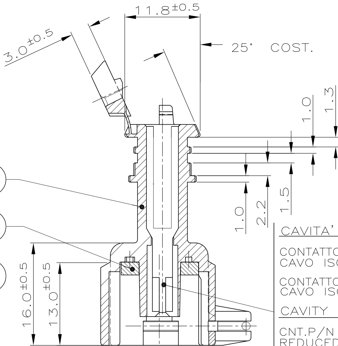
SEZIONE A-A (SECTION A-A)
