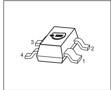
SOT143
