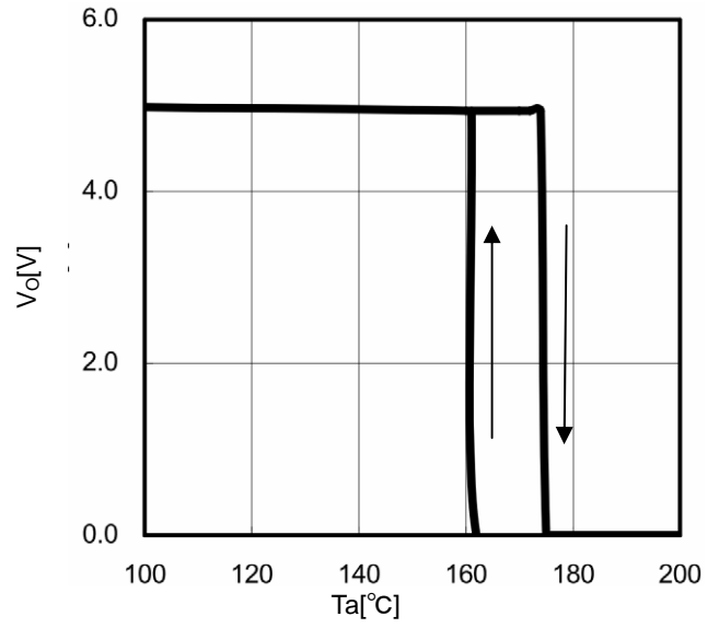
Fig.28 TSD (Io=0mA)
