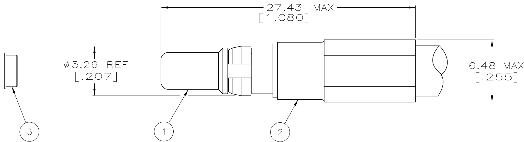
VIEW Y
