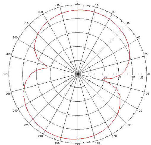
E-PLANE
