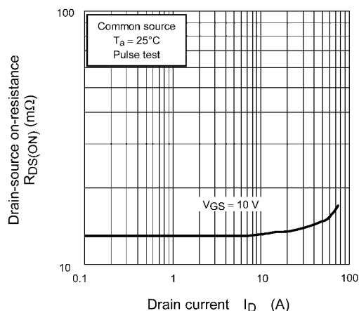
Fig. 8.6 R_{DS(ON)} - I_D
