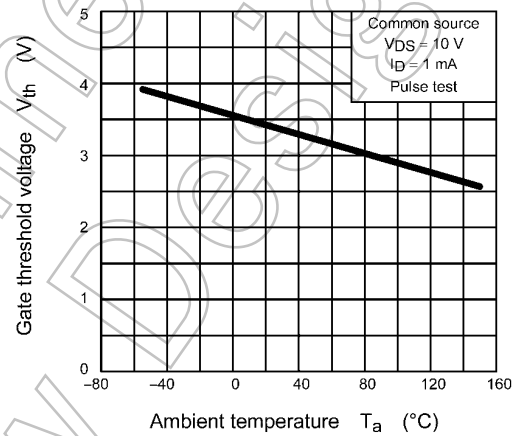
Fig. 8.10 V_{th} - T_a
