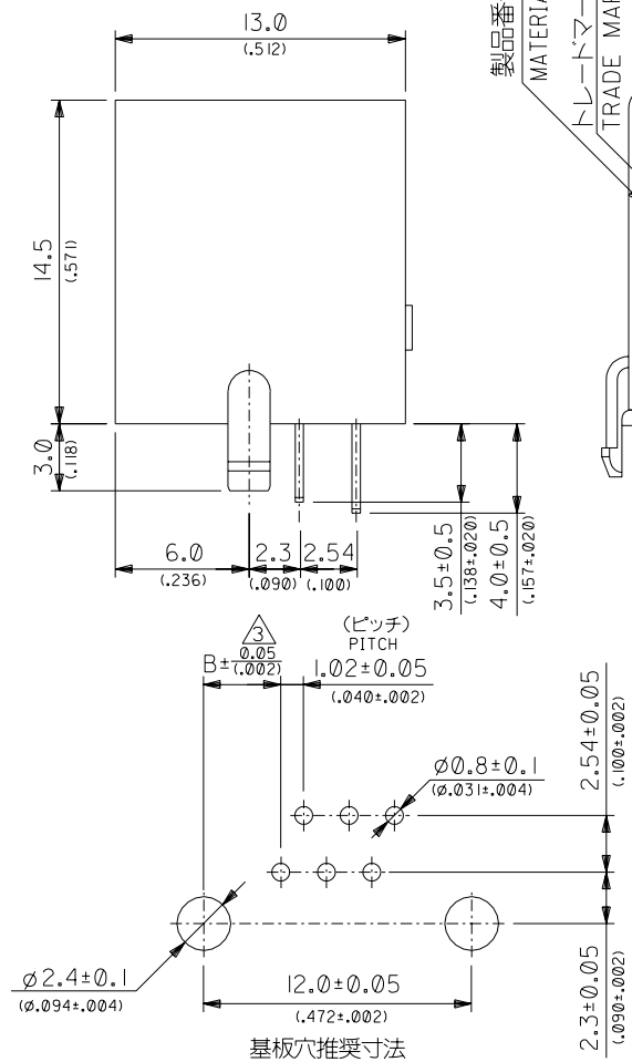
基板穴推奨寸法 RECOMMENDED P.C.B. LAYOUT (ジャック取付け側) (JACK ASS'Y SIDE)
