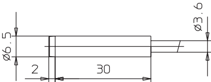
E2EL-C2M□ 2M
