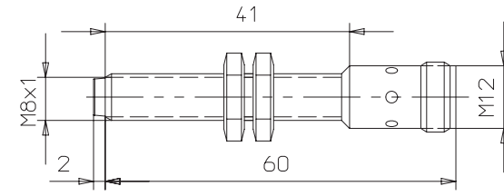
E2EL-X2M□-M1L
