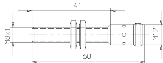
E2EL-X1R5□-M1L
