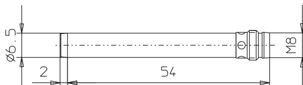
E2EL-X2M□-M3
