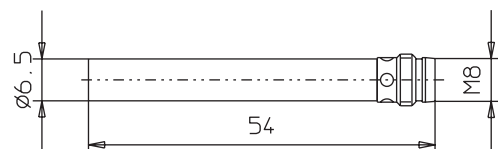
E2EL-C1R5□-M3L
