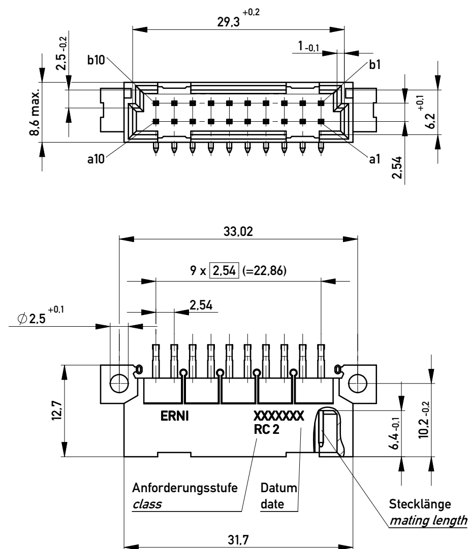
Bestückungsplan / contact layout
