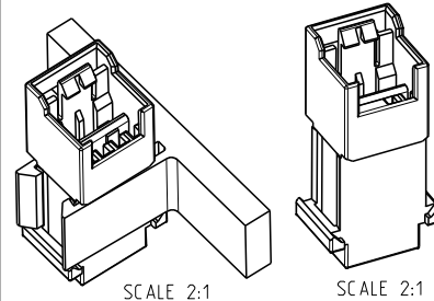
VIEW: ASSEMBLY WITH CONTACT Darstellung: Assembly mit Kontakt
