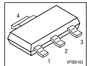
PG-SOT223
