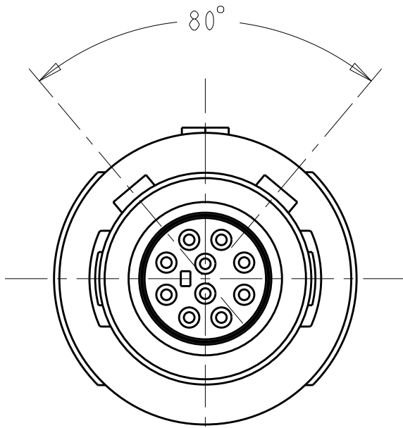
80° KEYING SCALE 4:1
