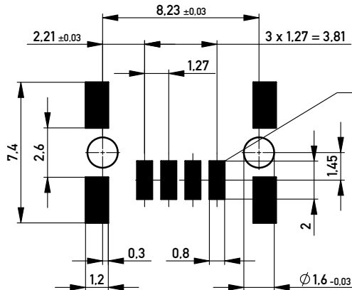
Leiterplatten-Layout für SMT PCB-Layout for SMT
