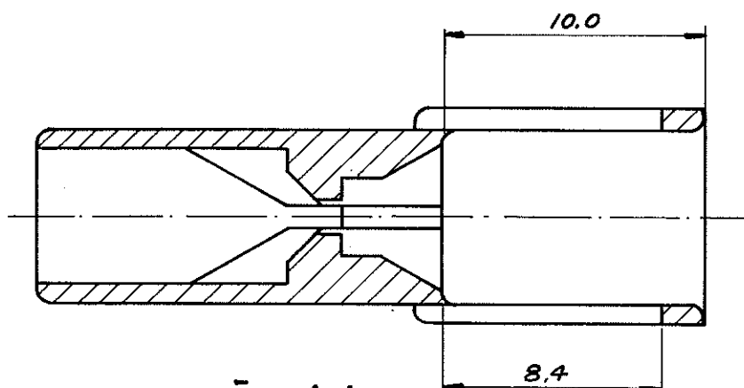
SECCÃO A-A
