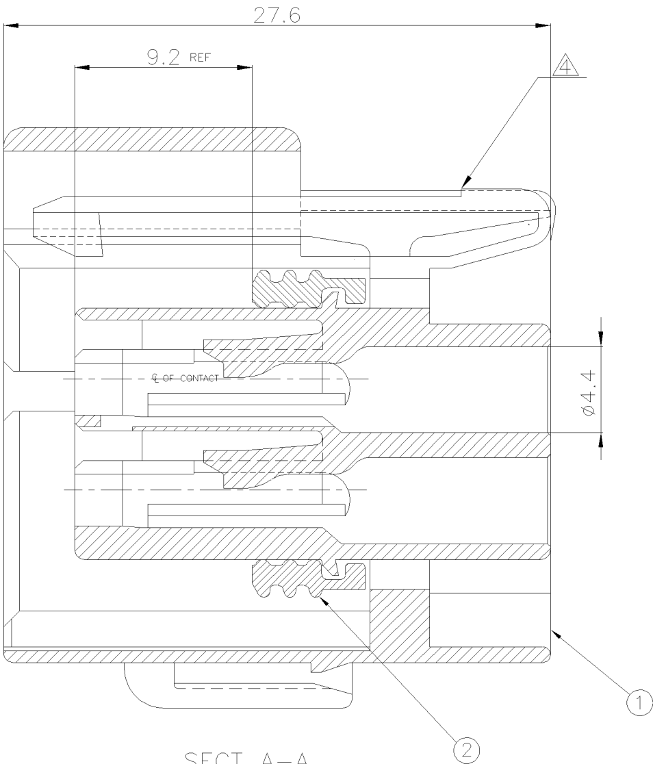
SECT A-A
