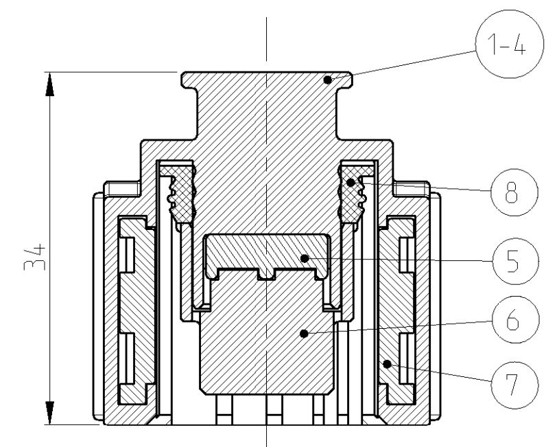
SECTION A-A Schnitt
